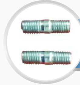
STUD (M10*33)
